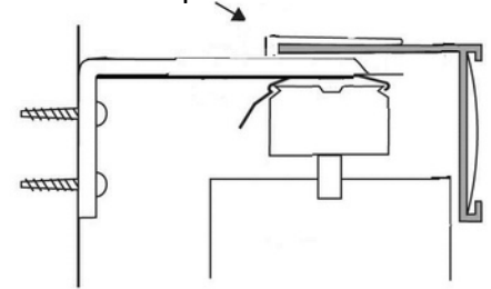
Valance Clip
